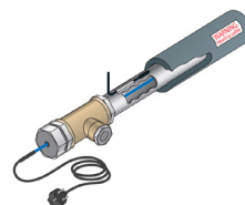
Montavimas vandens vamzdžių viduje
