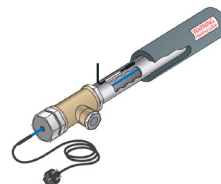
Монтаж внутри водопроводной трубы
