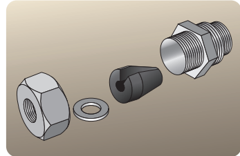
3/4 col. + 1 col. vamzdžio tvirtinimo detalė, skirta „DEVIpipeline™ 10 V3“ (140F0956)
