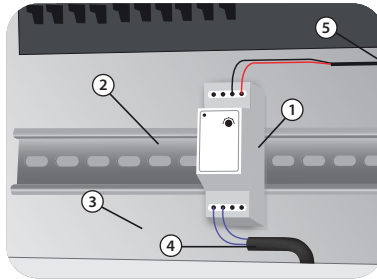
1 — контроллер; 2 — DIN-рейка; 3 — электрический шкаф; 4 — подключение холодного провода; 5 — подключение датчика
