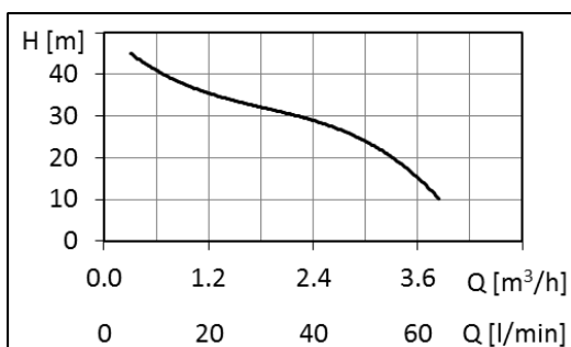
Sūkņa darba līkne
